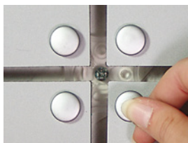
fissaggio di pannelli con il distanziale zigrinato fixxo. panelbefestigung mit fixxo klücksystem. panel mounting with fixxo click-in.
