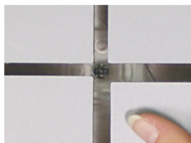
fissaggio invisibile di pannelli con ghost oppure con fixxo (FIXXK16WEFL). unsichtbare panelbefestigung mit ghost oder fixxo (FIXXK16WEFL). invisible panel mounting with ghost or fixxo (FIXXK16WEFL).
