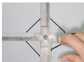
fissaggio dei pannelli con anellini di silicone. panelbefestigung mit silikon-ringen. panel mounting with silicone oring.
