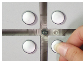
fissaggio di pannelli con il distanziale zigrinato fixxo. panelbefestigung mit fixxo klicksystem. panel mounting with fixxo click-in.
